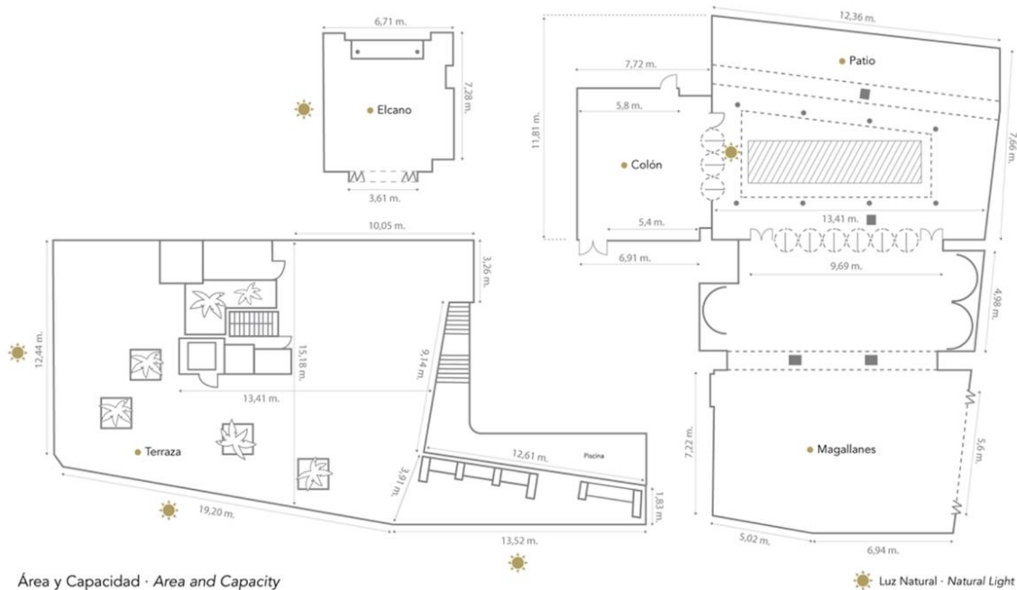
Àrea y Capacidad · Area and Capacity
